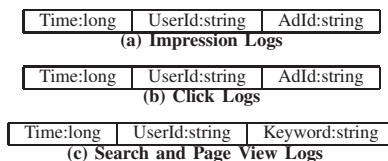
Fig. 1. Schemas for BT data.
